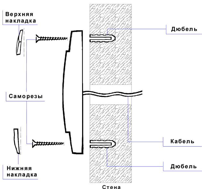
Рисунок 1. Крепление контроллера.
