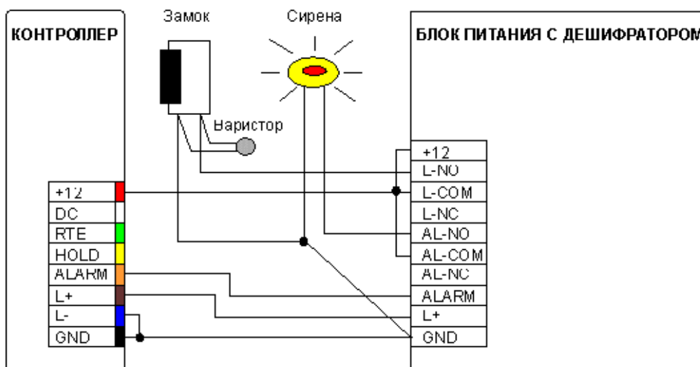
Рисунок 5. Управление замком и сиреной через дешифратор
