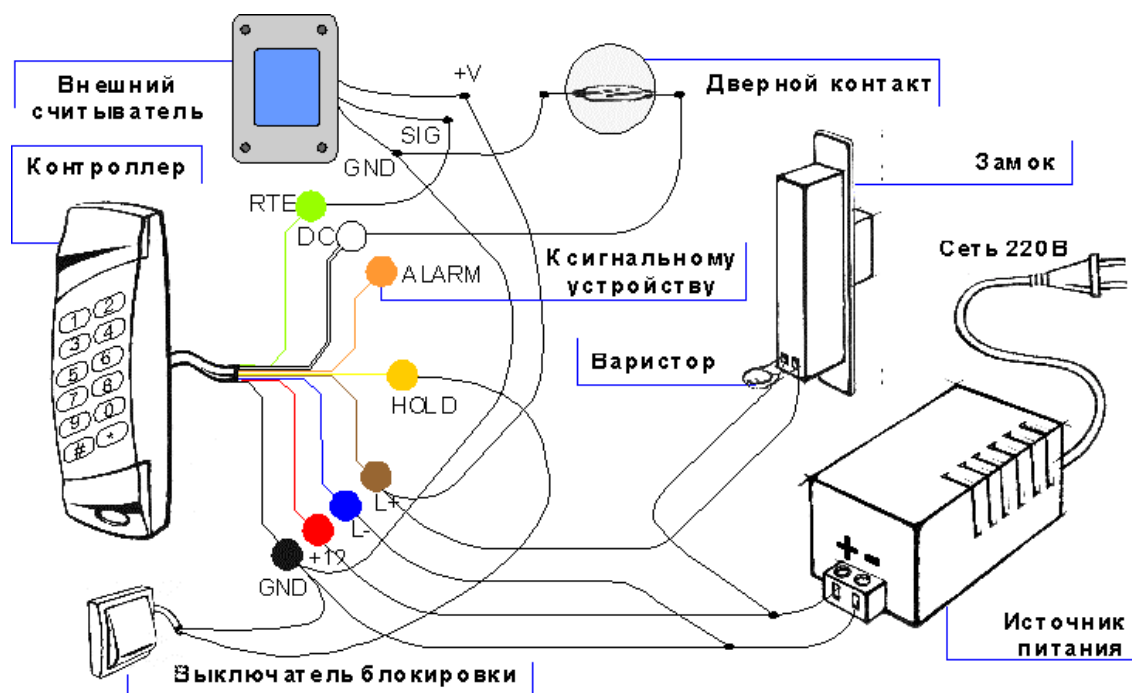
Рисунок 4. Подключение внешнего считывателя.
